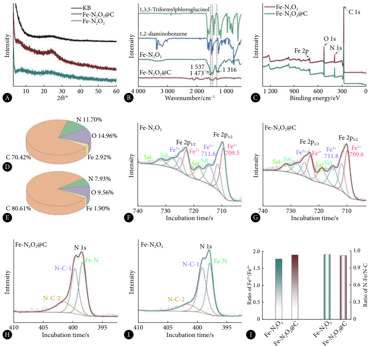
图 3 \text{Fe-N}_2\text{O}_2 和 \text{Fe-N}_2\text{O}_2\text{@C} 的配位结构分析
